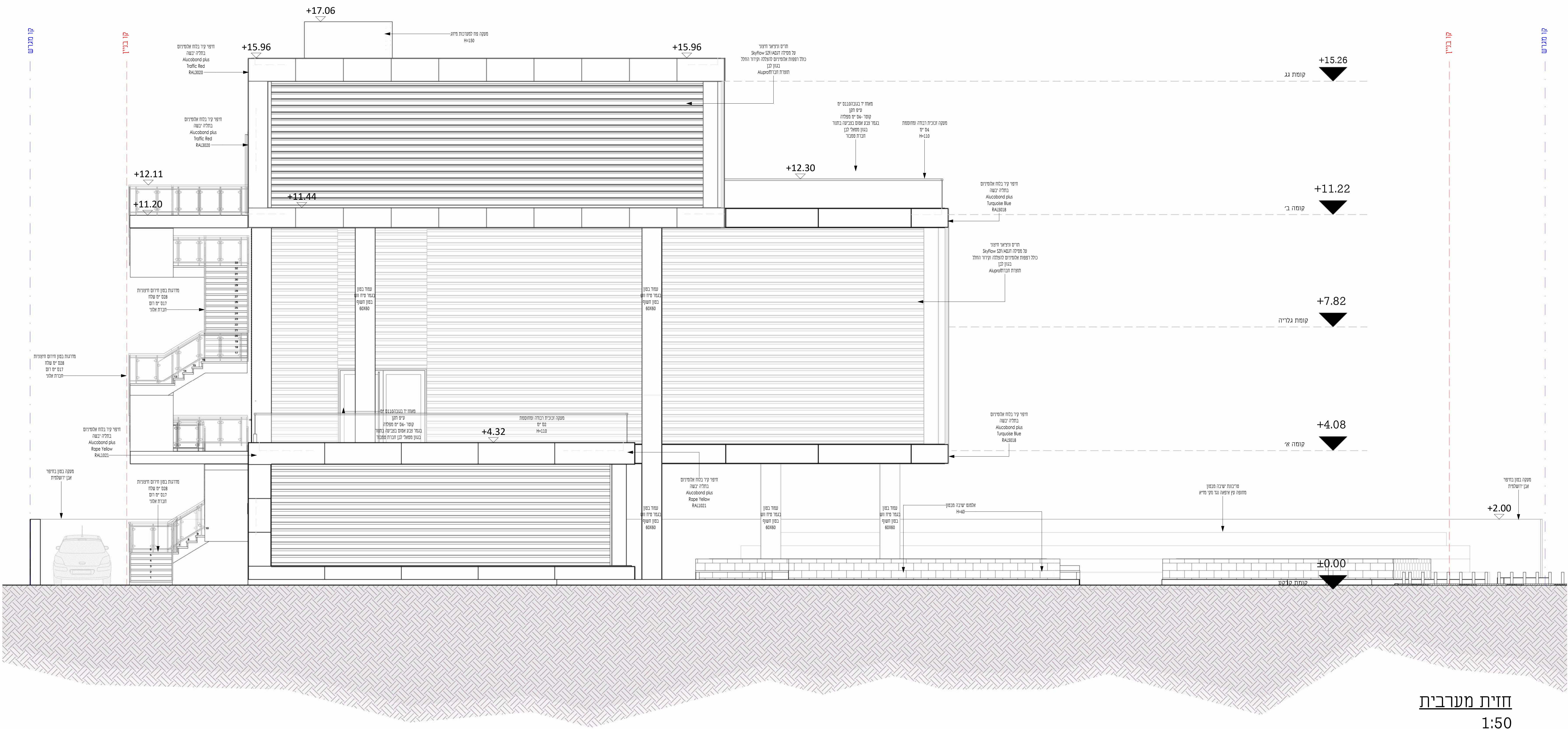
חזית דרומית 1:50
