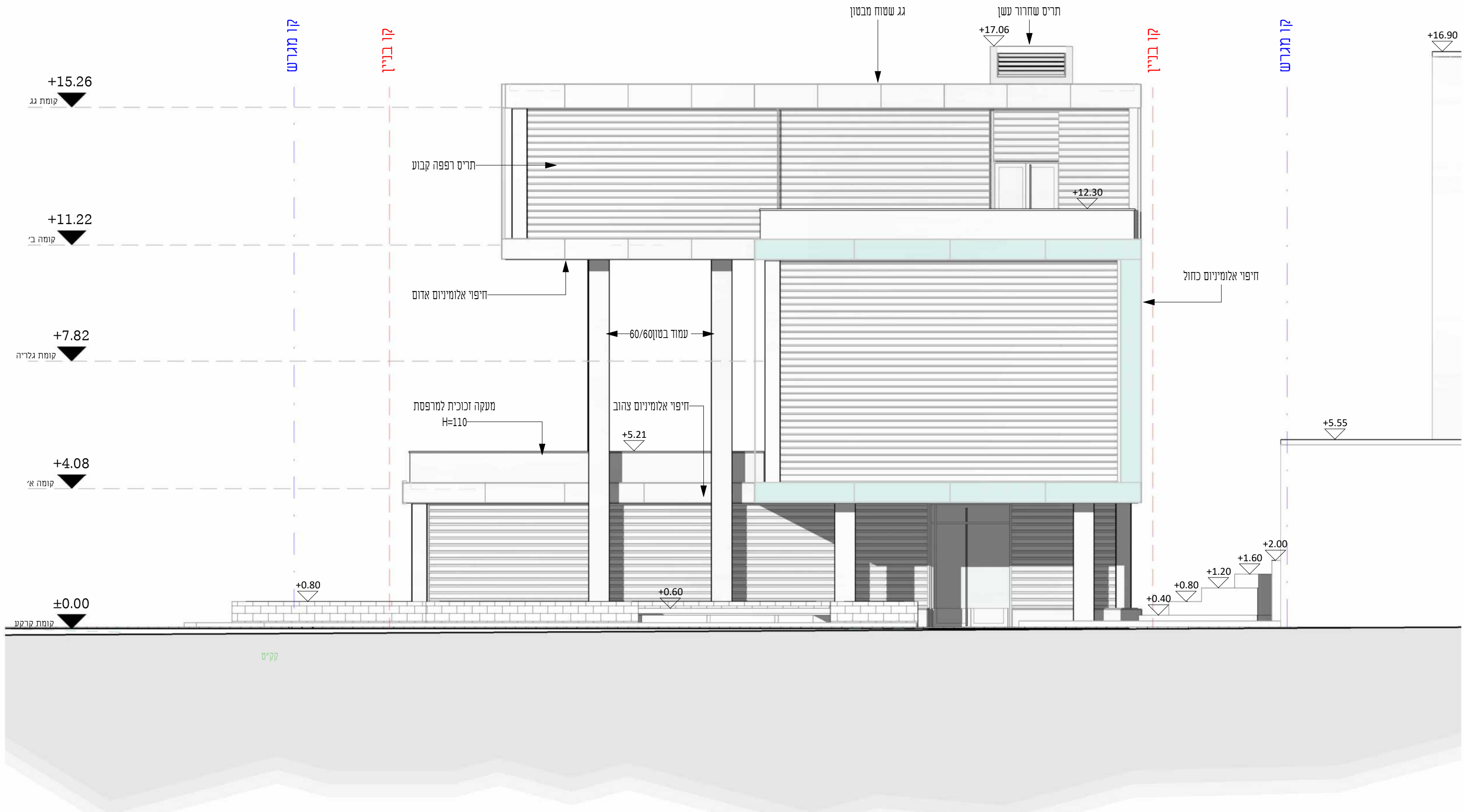
חזית דרומית 1:100
