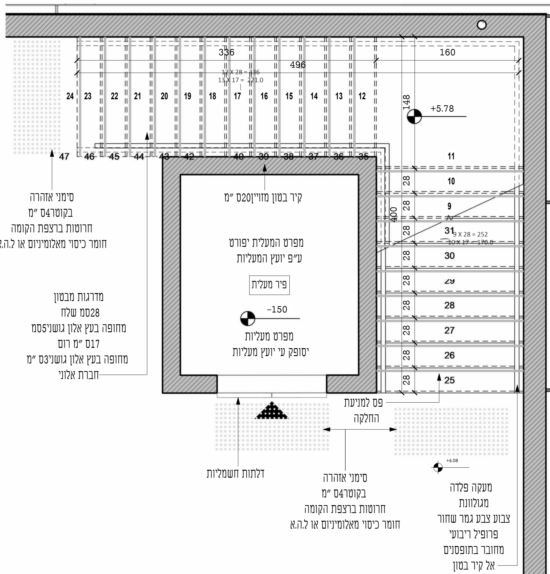
תוכנית מדרגות קומה א' 1:25
