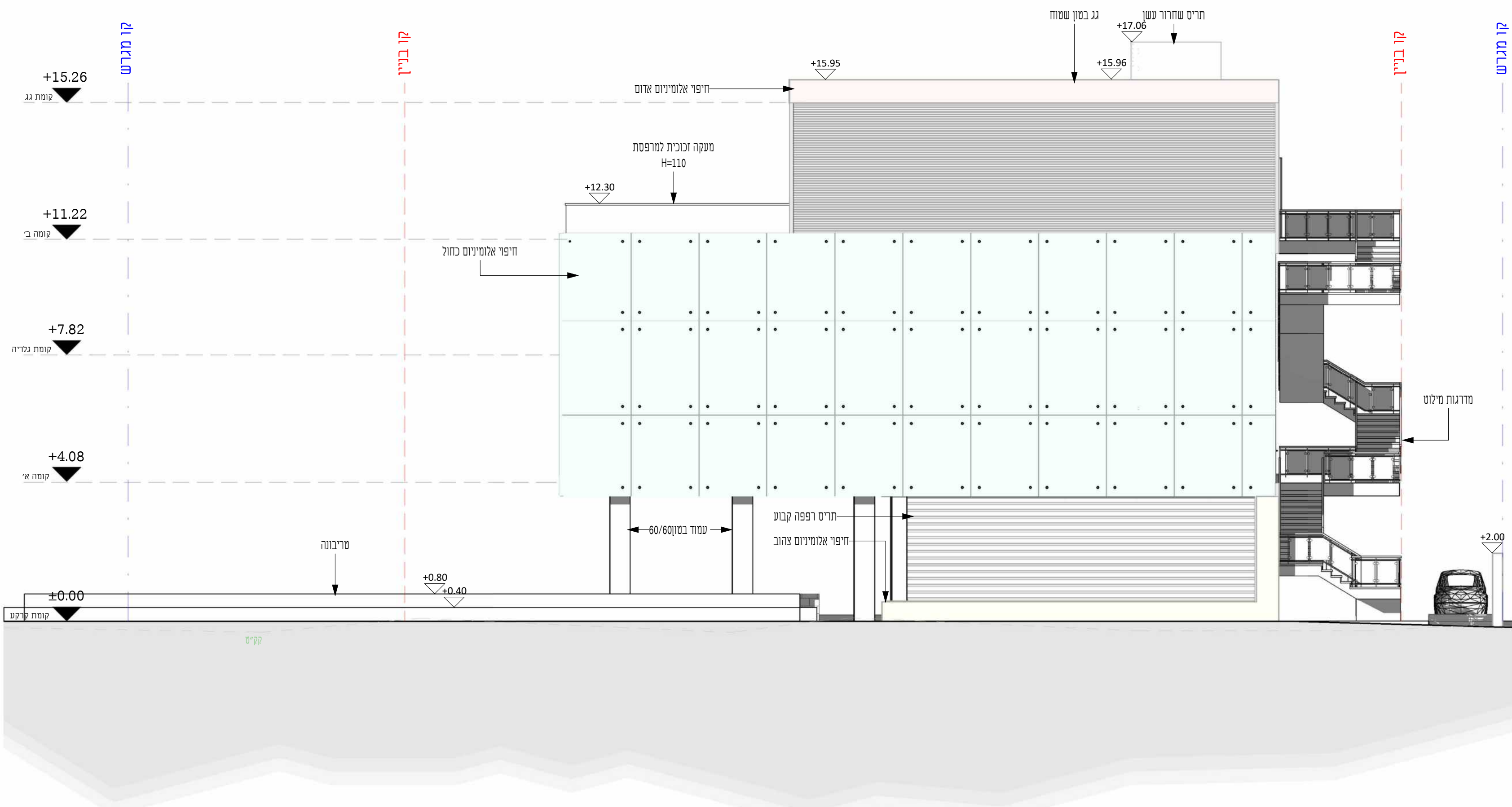
חזית מזרחית 1:100
