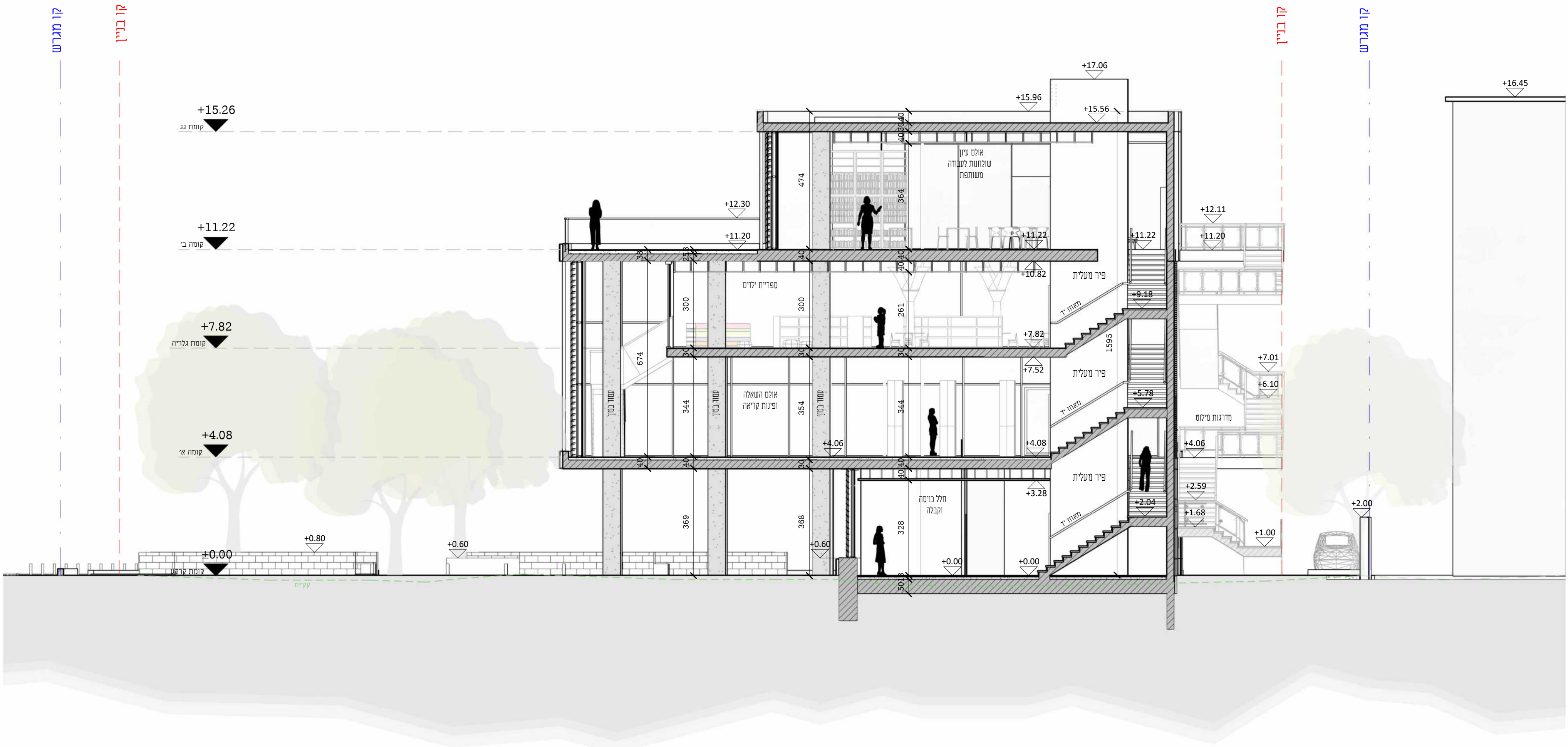
חתך ב-ב' להמחשה 1:100
