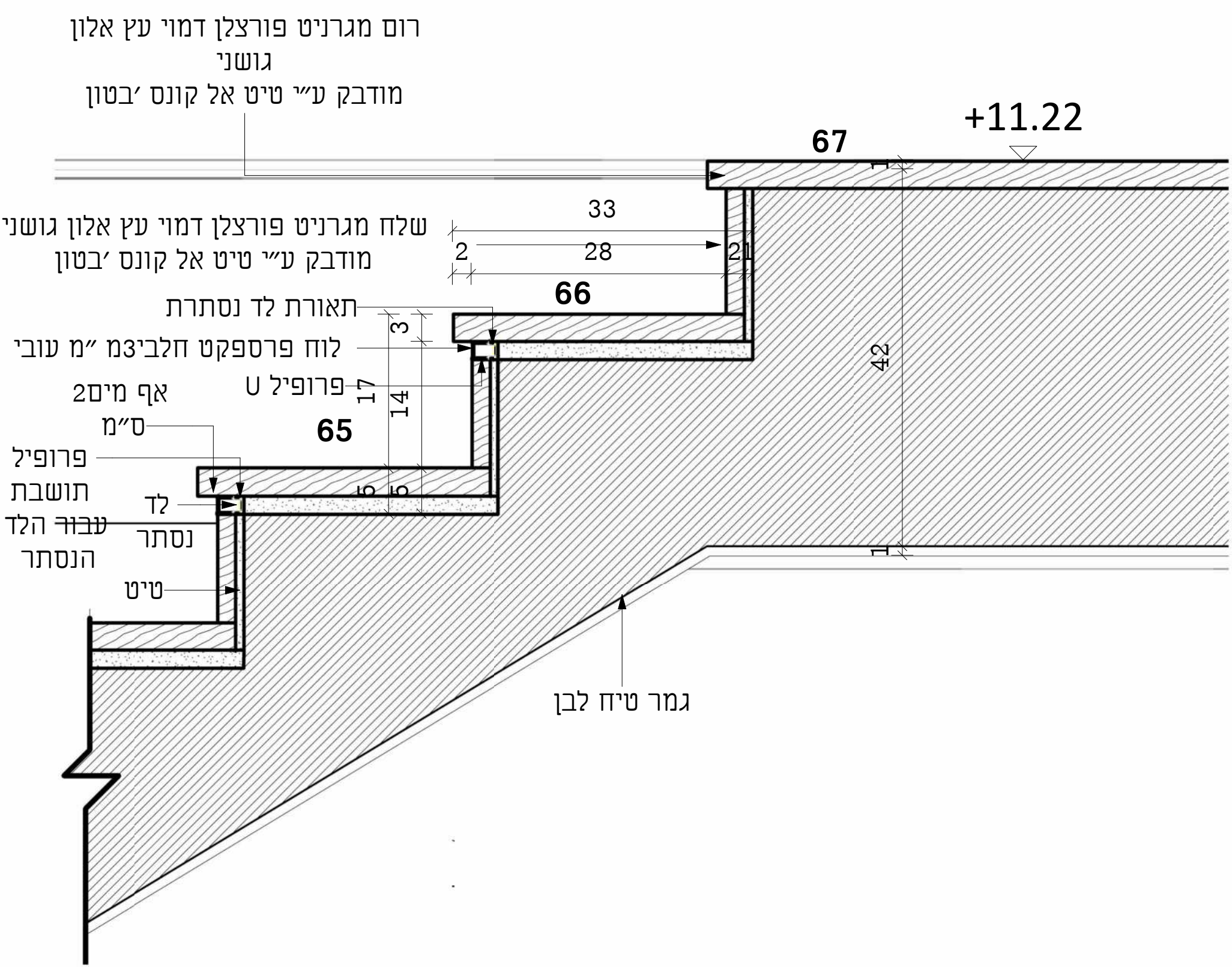
פרט מדרגה אחרונה 1:5
