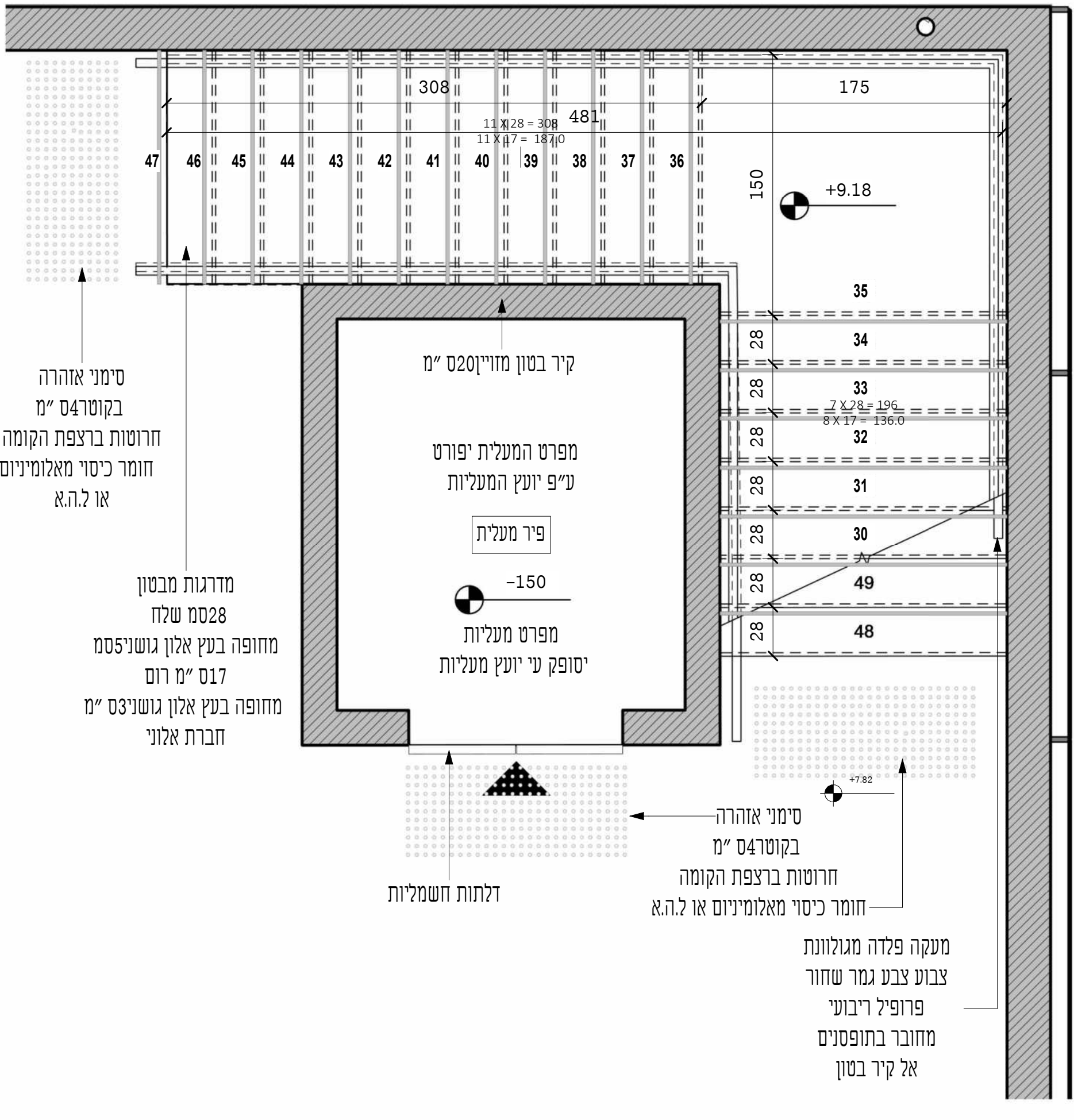
תוכנית מדרגות קומת גלריה 1:25
