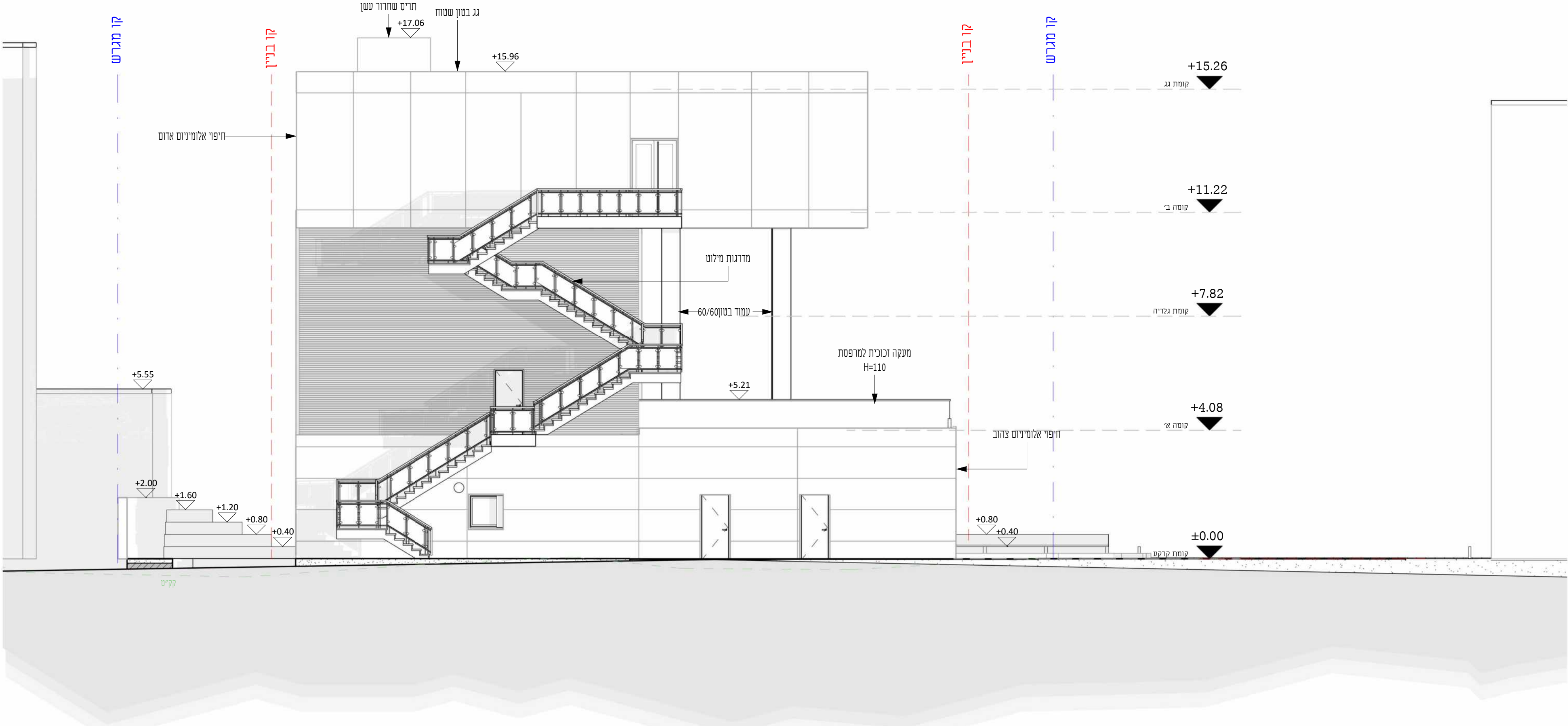
חזית צפונית 1:100
