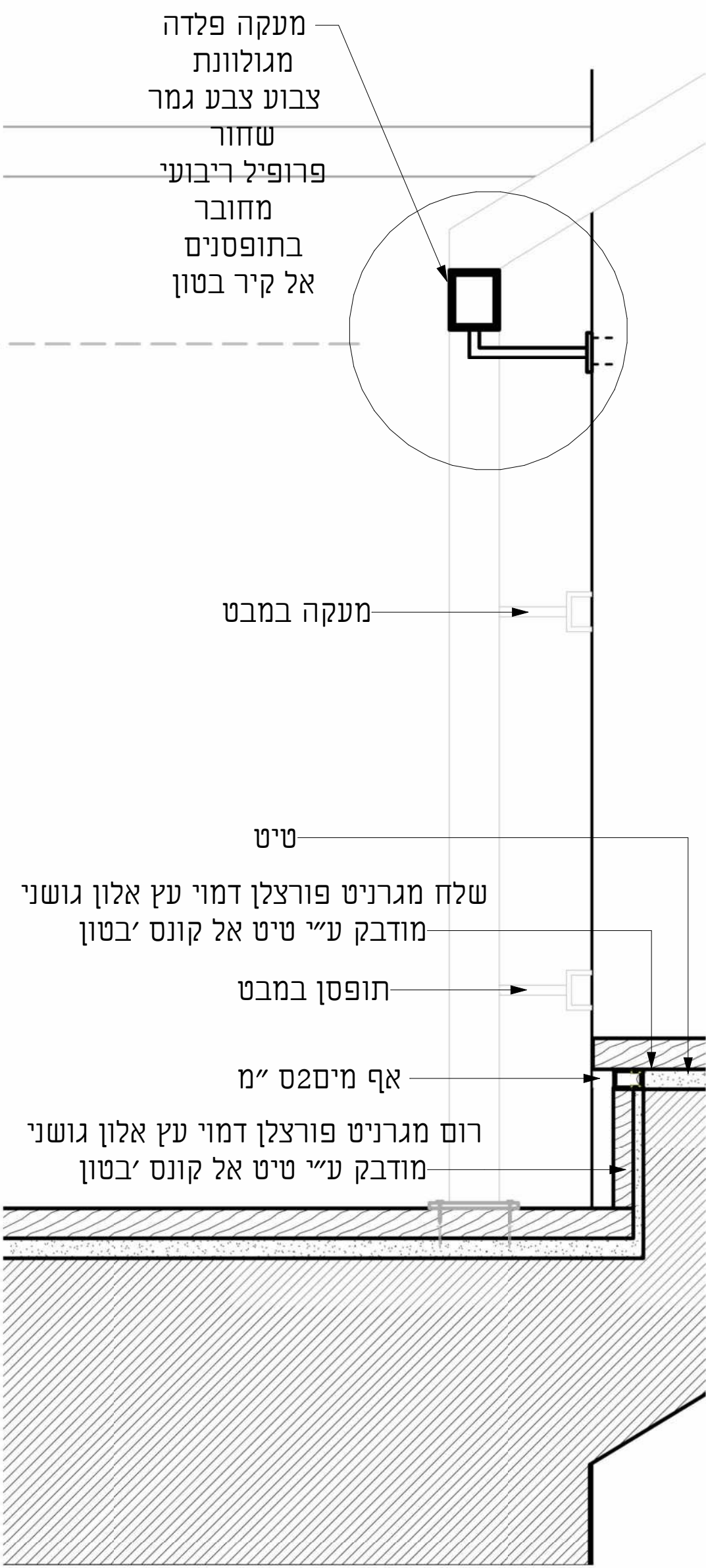
פרט מעקה 1:5
