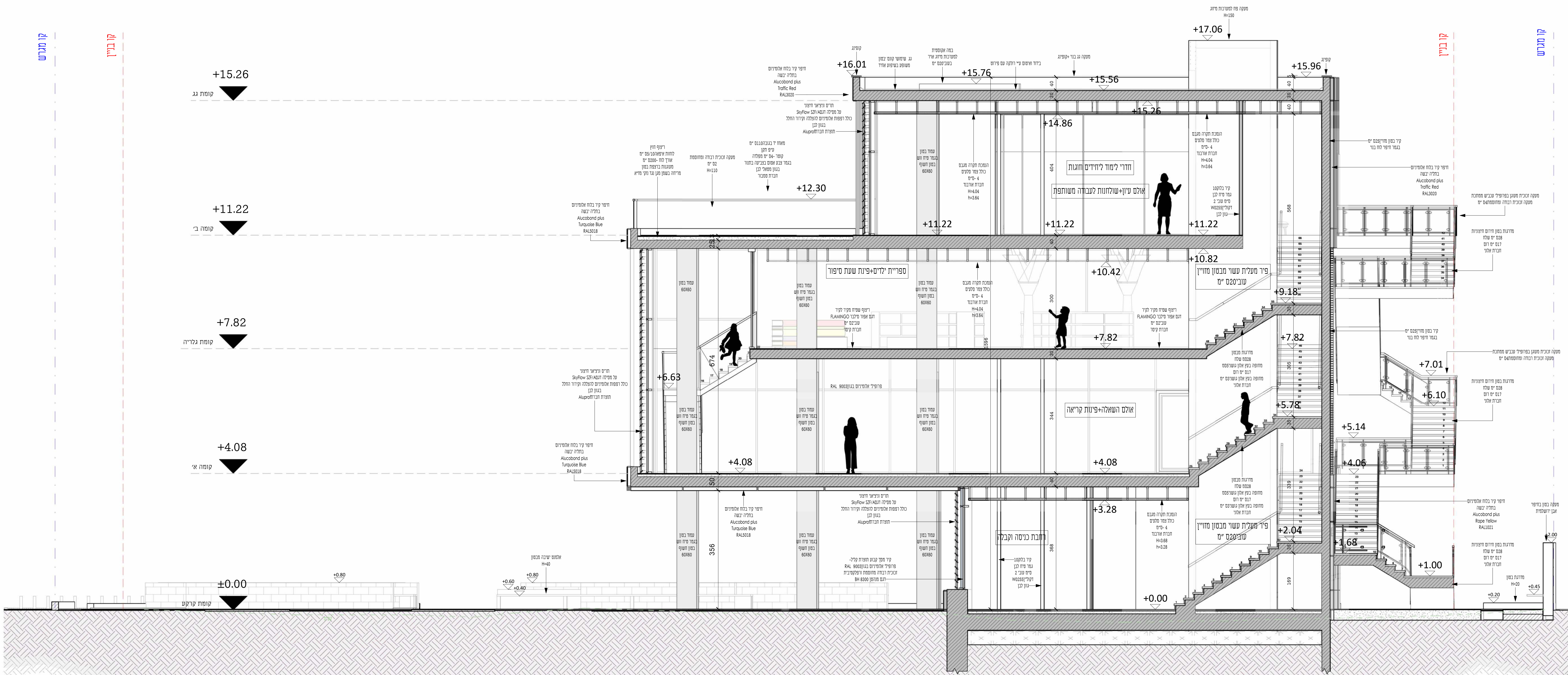
חתך ב'-ב' 1:50
