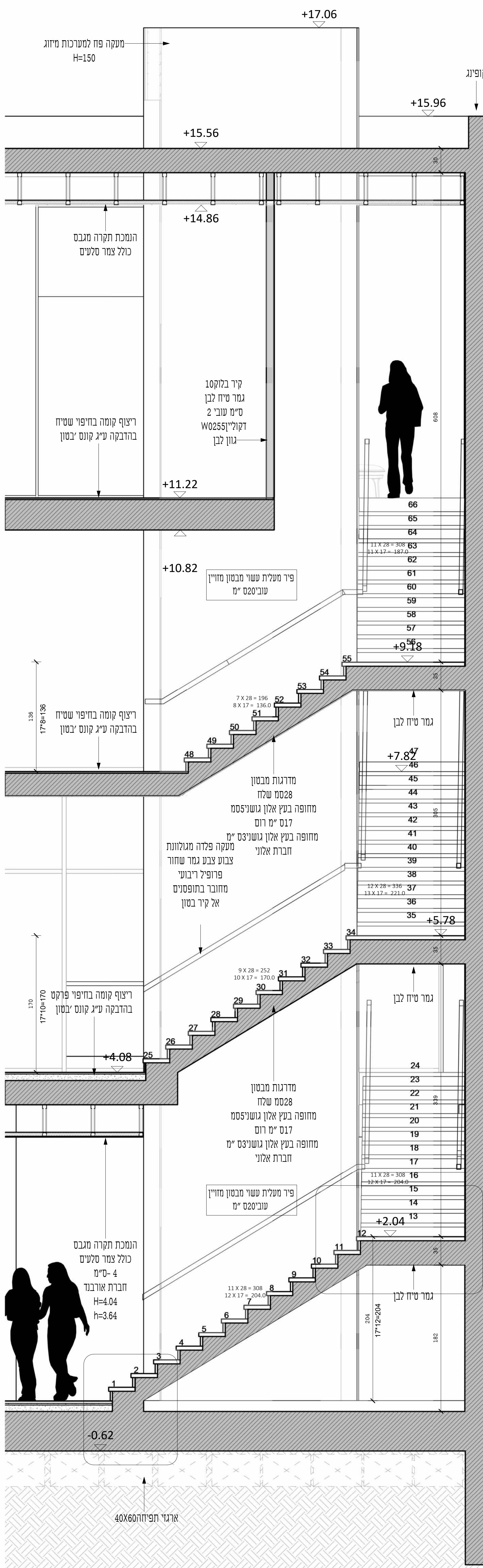
חתך מדרגות ב-ב' 1:25
