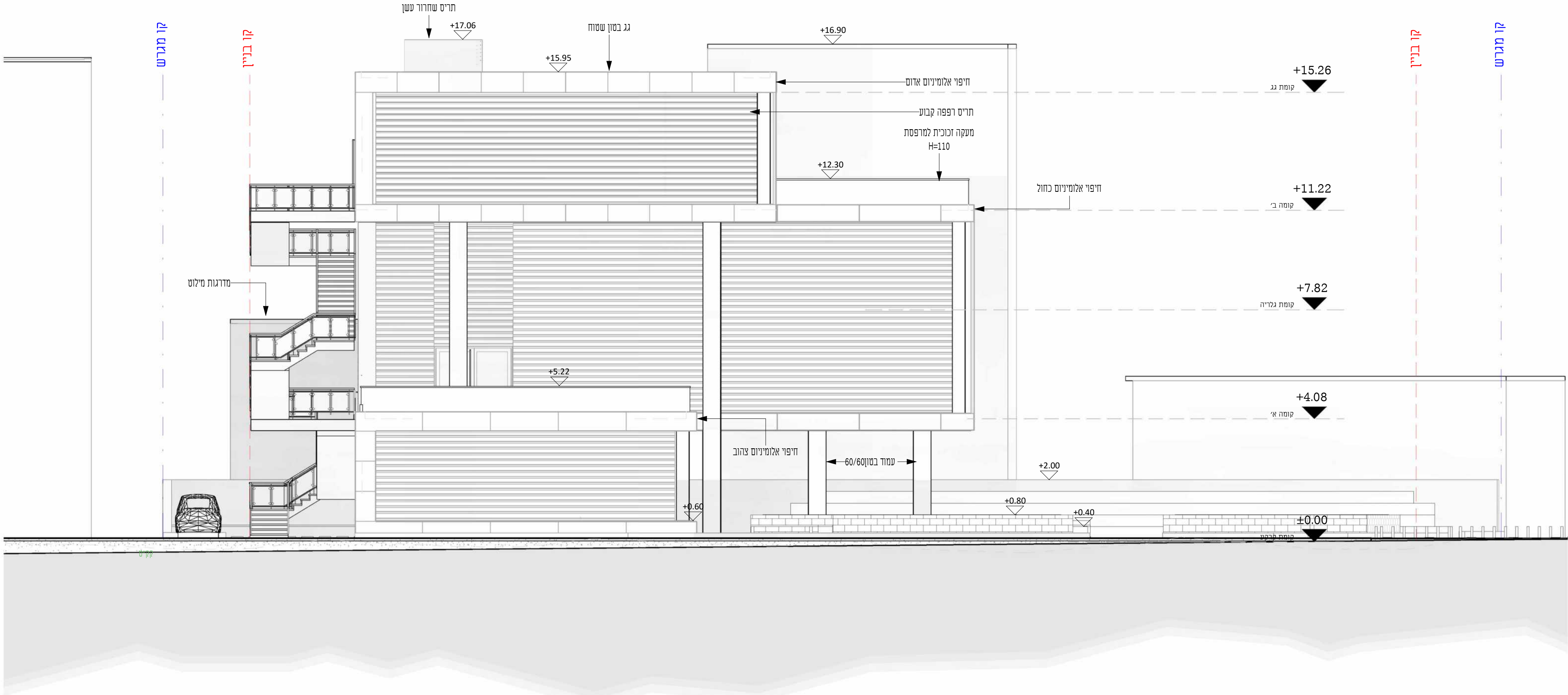
חזית מערבית 1:100
