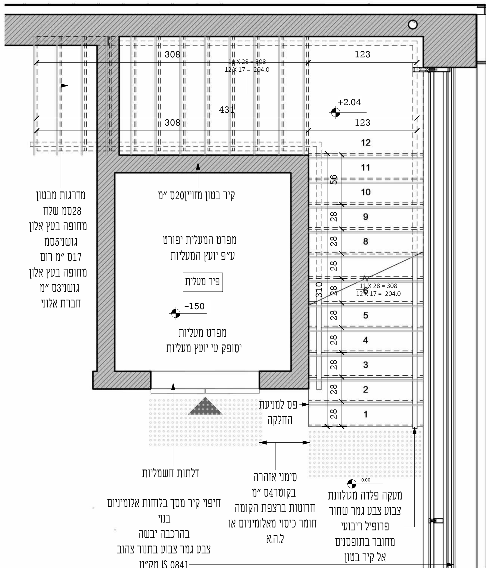
תוכנית מדרגות קומת קרקע 1:25
