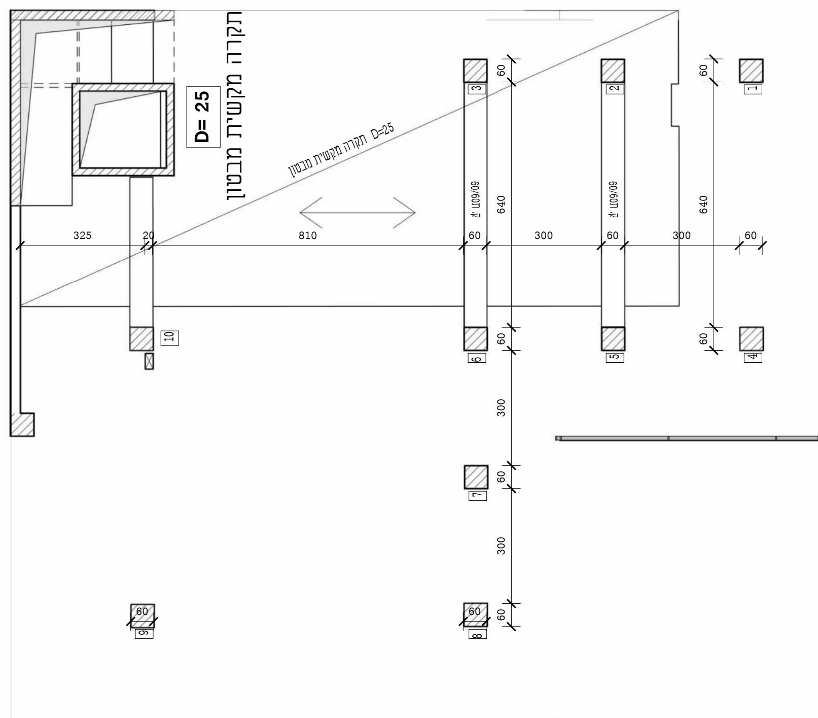
תקרה במפלס 7.82 1:100
