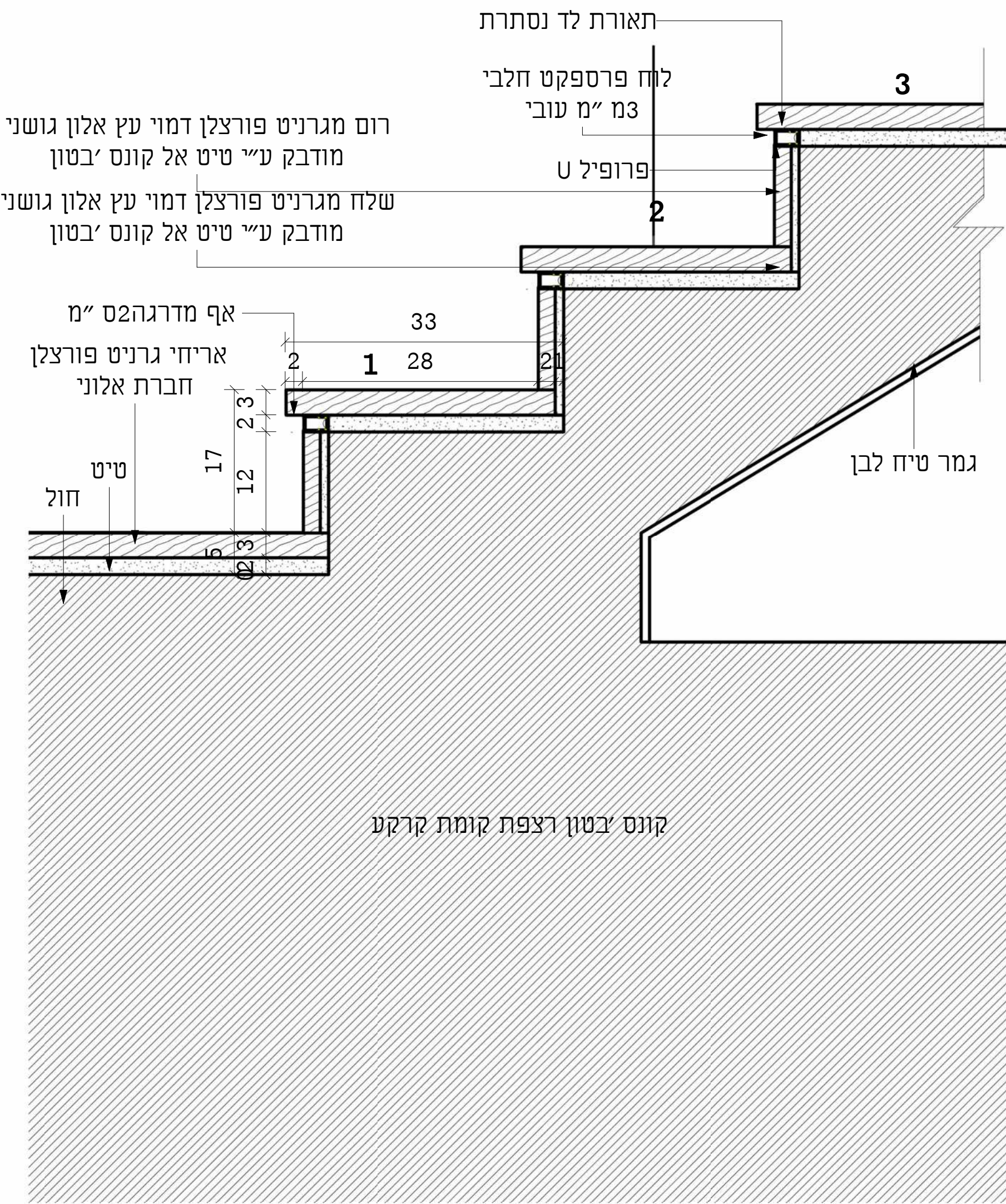
פרט מדרגה ראשונה 1:5
