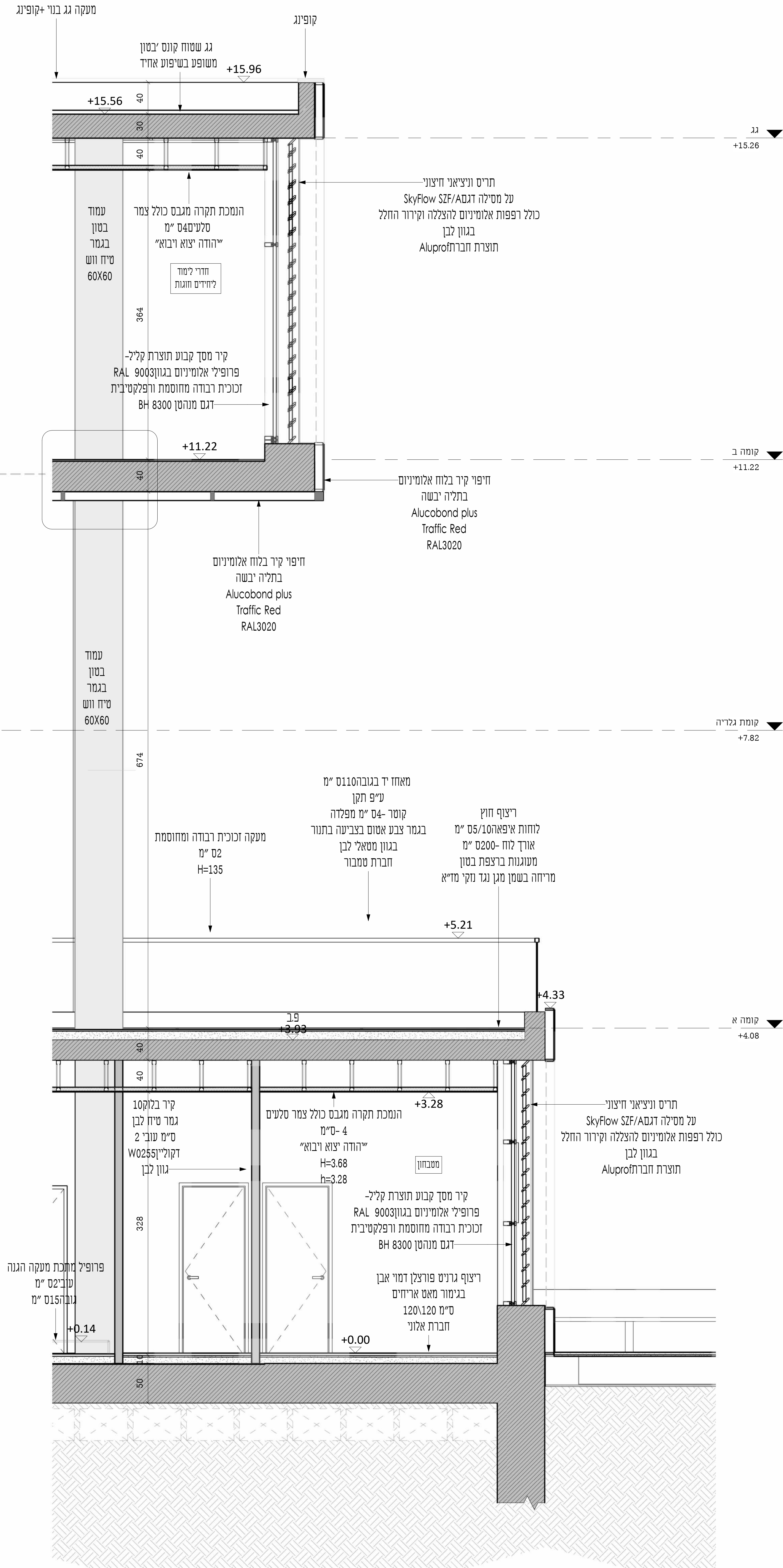
חיתך מעטפת 1:25
