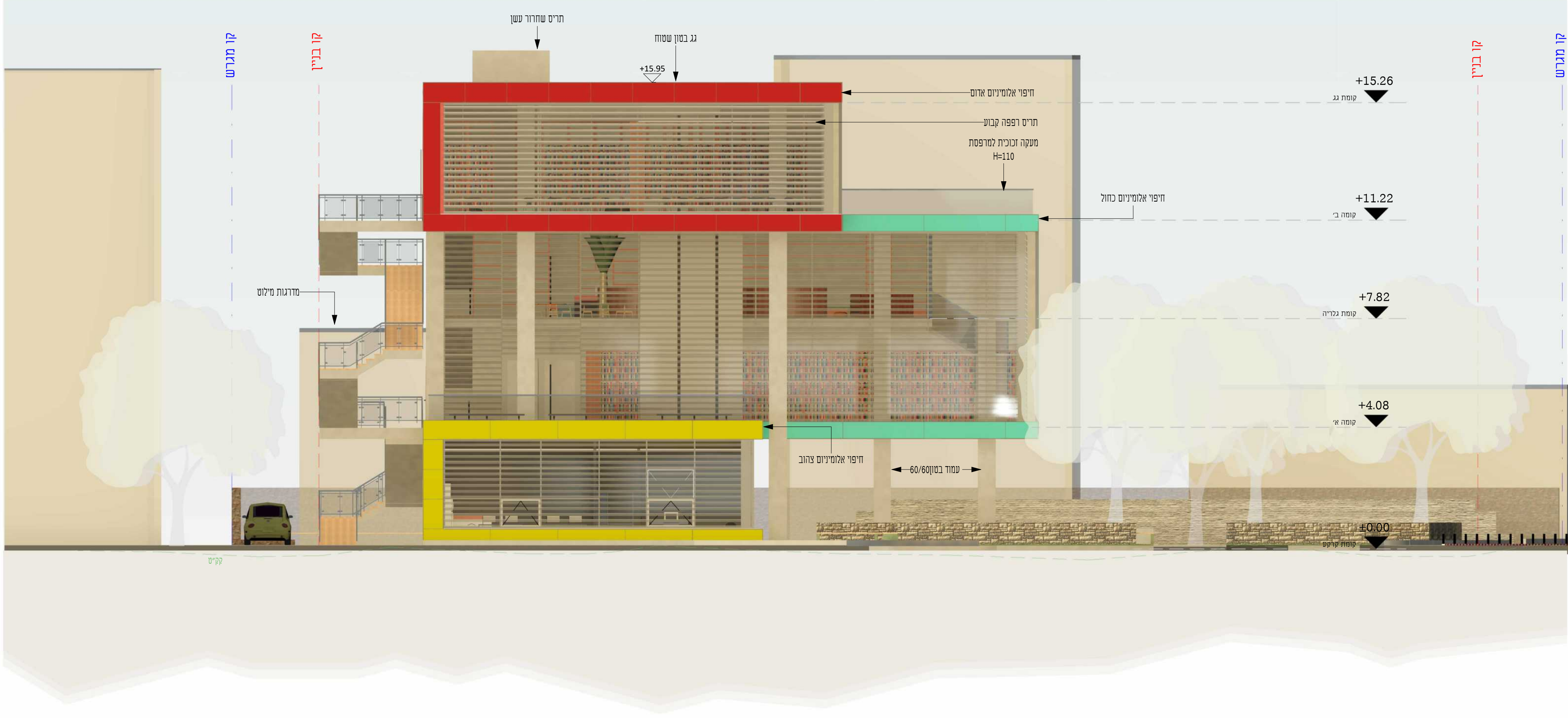
חזית מערבית להמחשה 1:100
