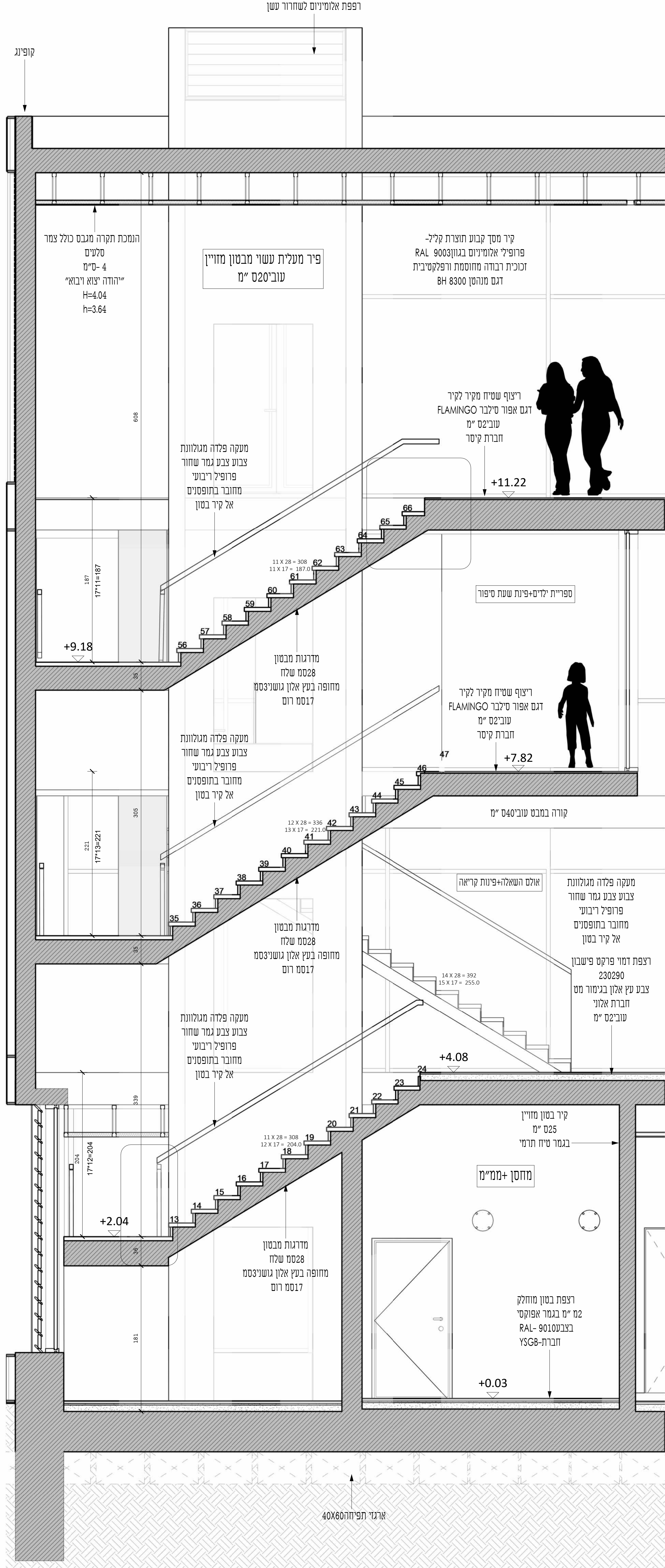
חתך מדרגות א-א' 1:25
