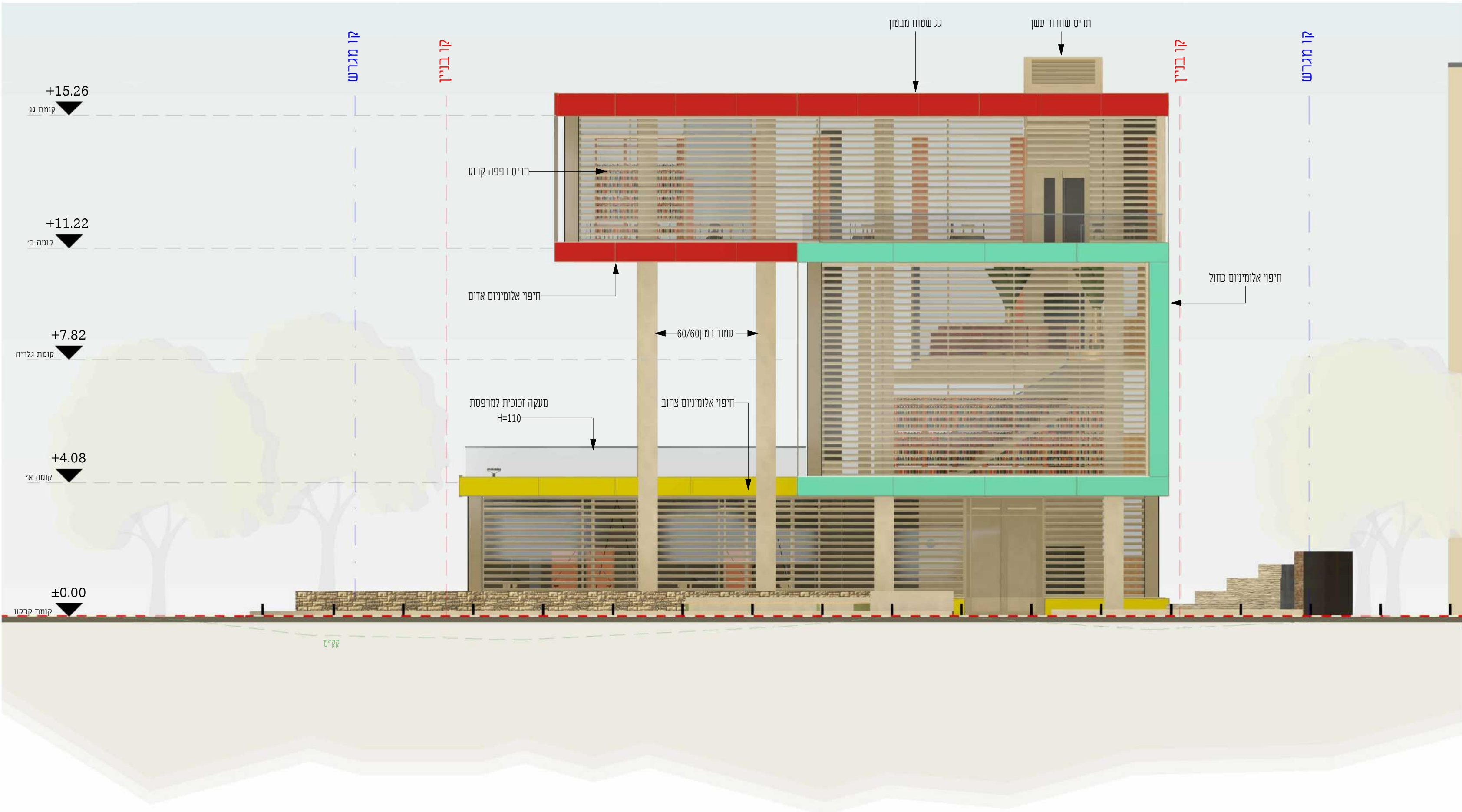
חזית דרומית להמחשה 1:100
