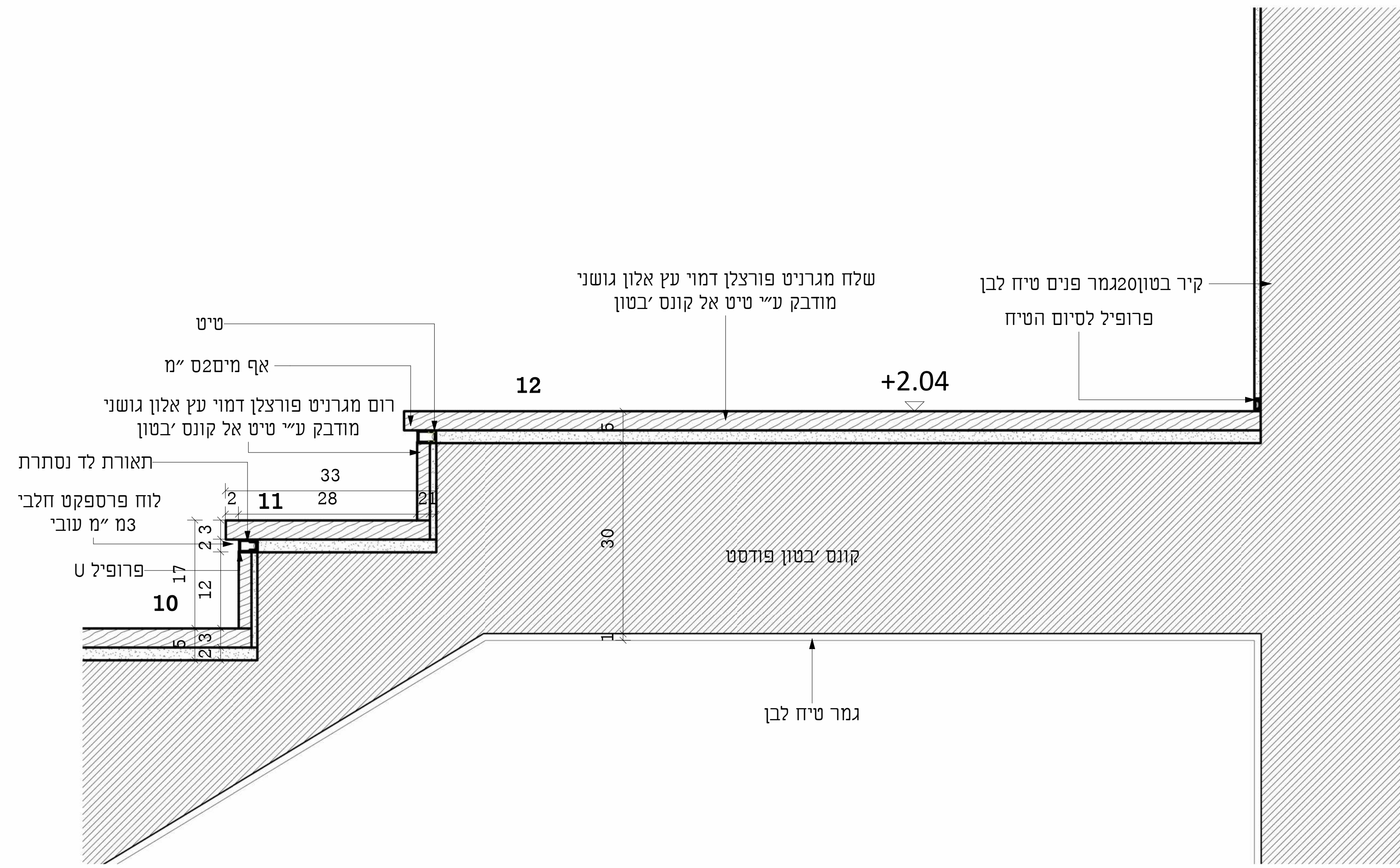
פרט פודסט 1:5
