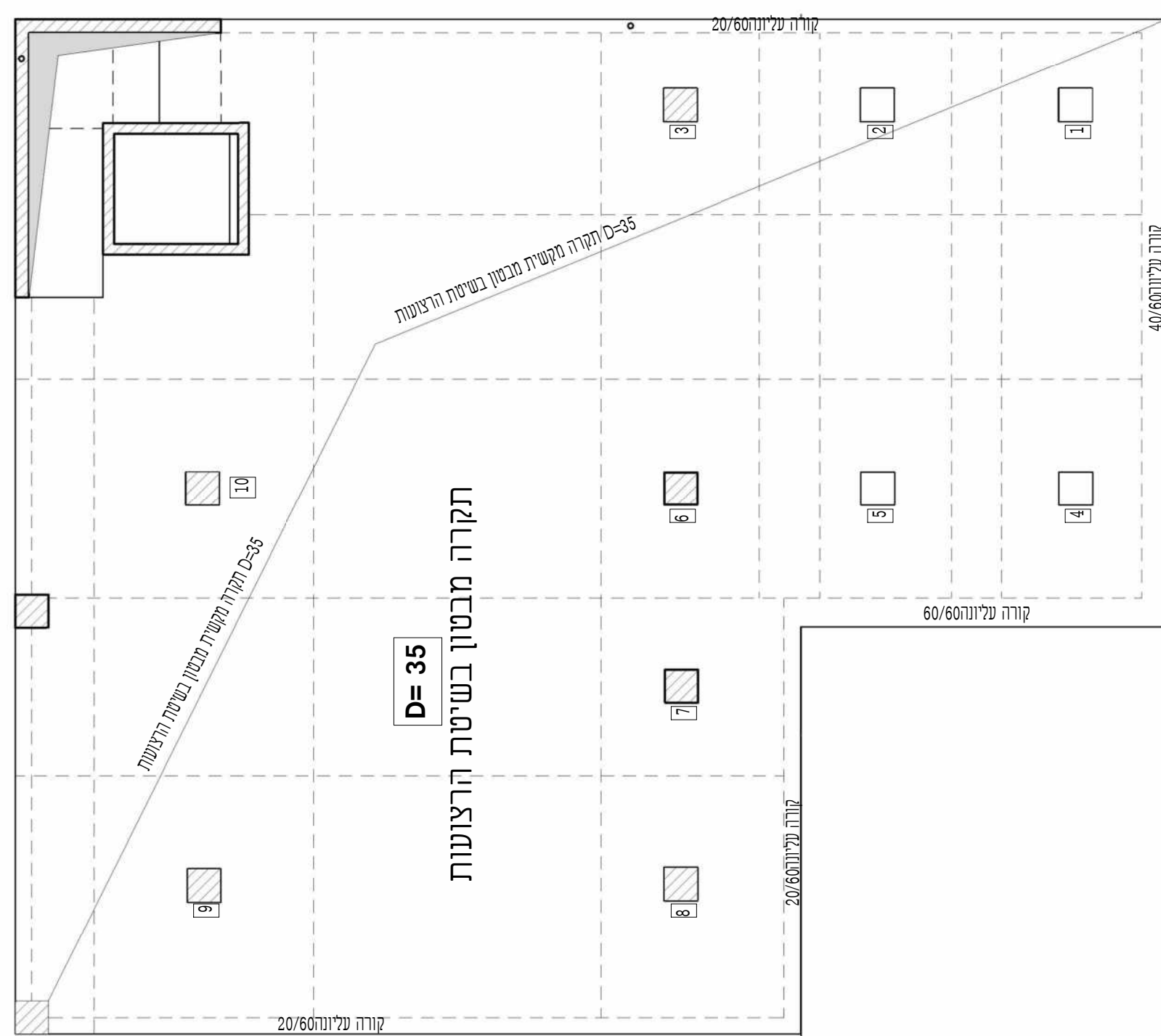
תקרה במפלס 11.22 1:100
