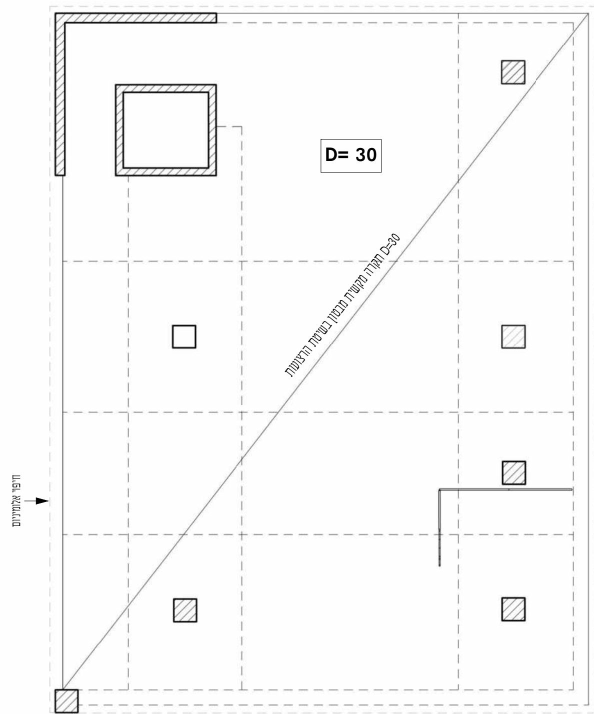
תקרה במפלס 15.56 1:100
