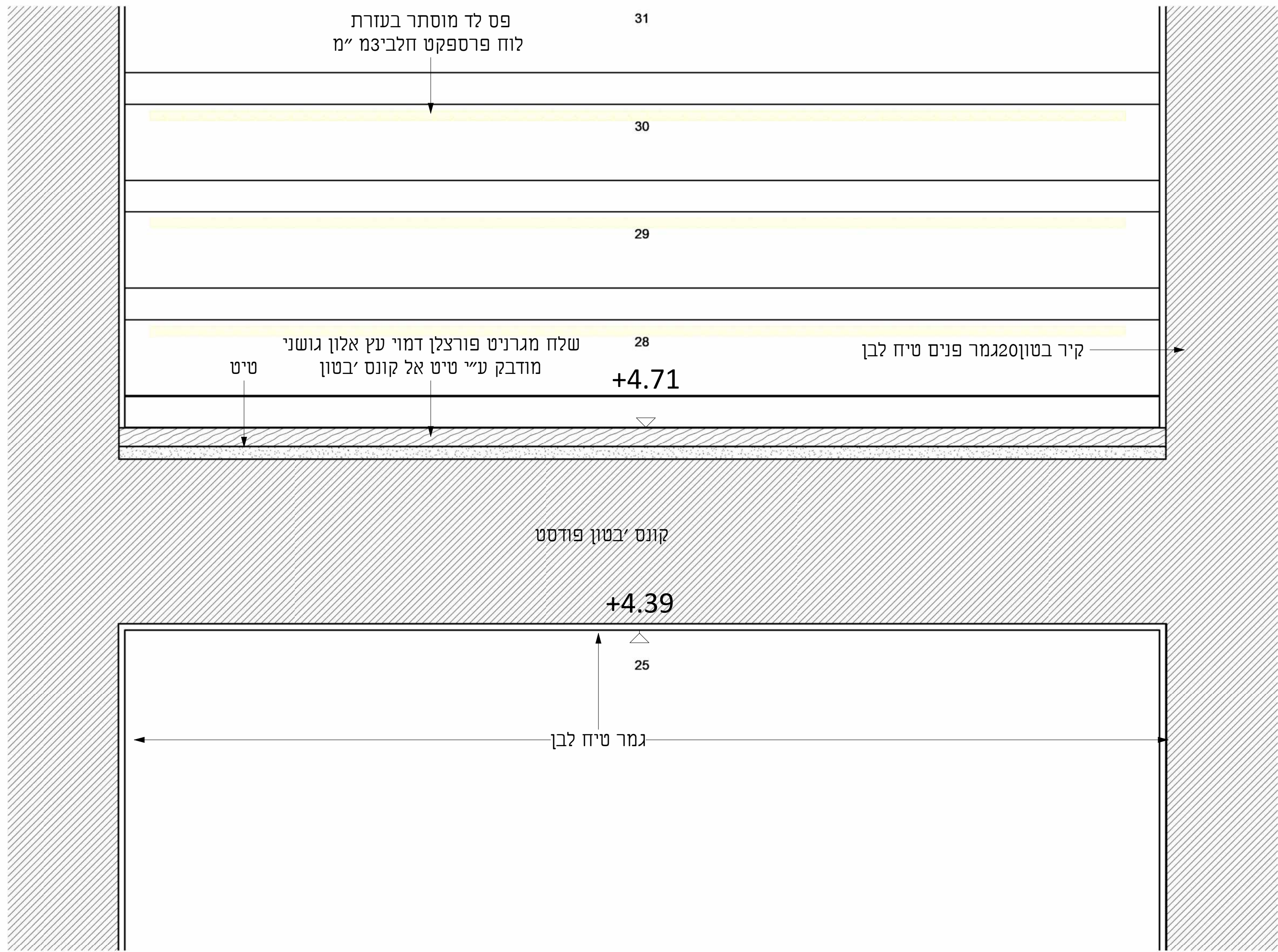
פרט מדרגה טיפוסית 1:5
