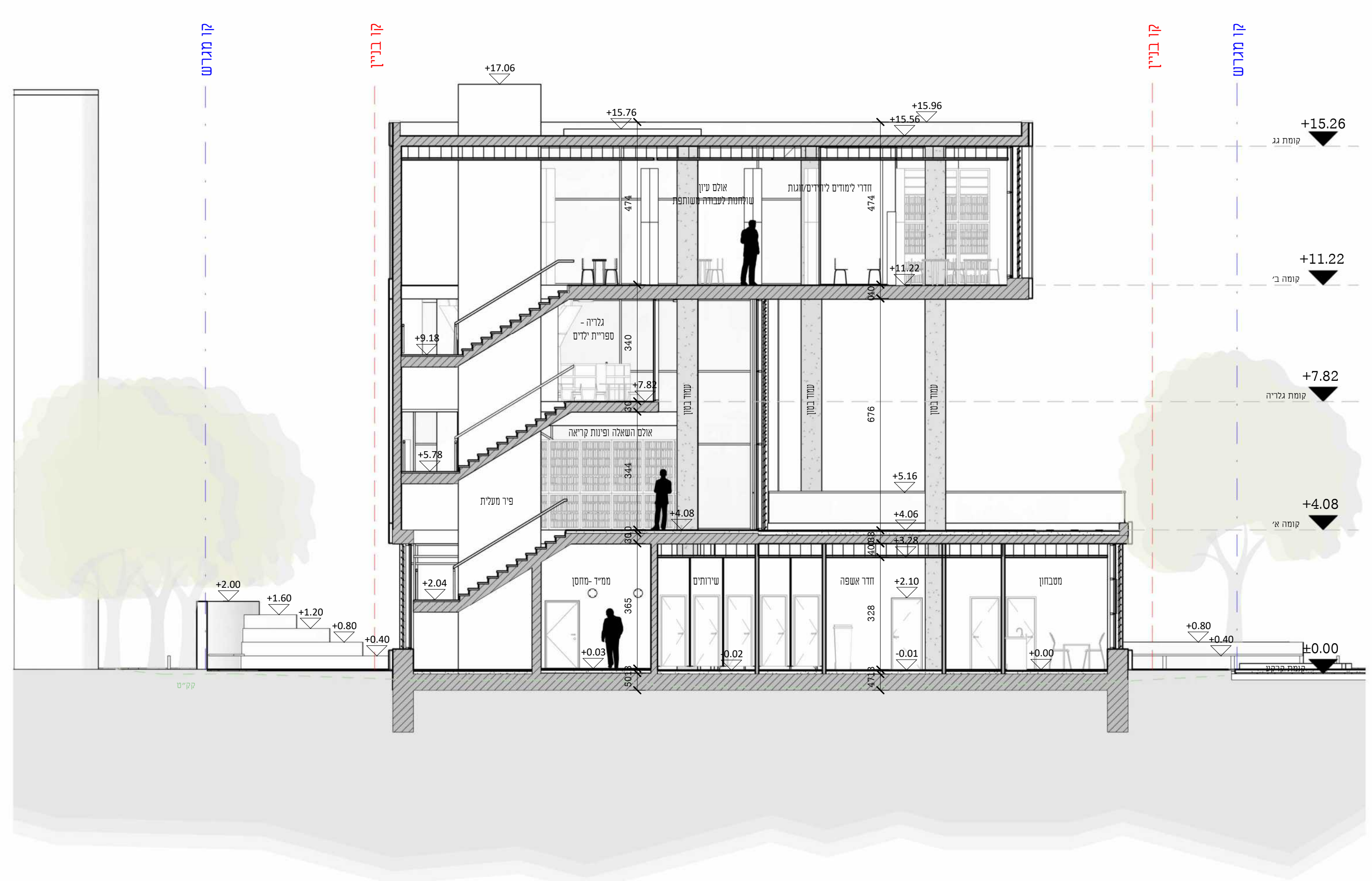
חתך א-א' להמחשה 1:100
