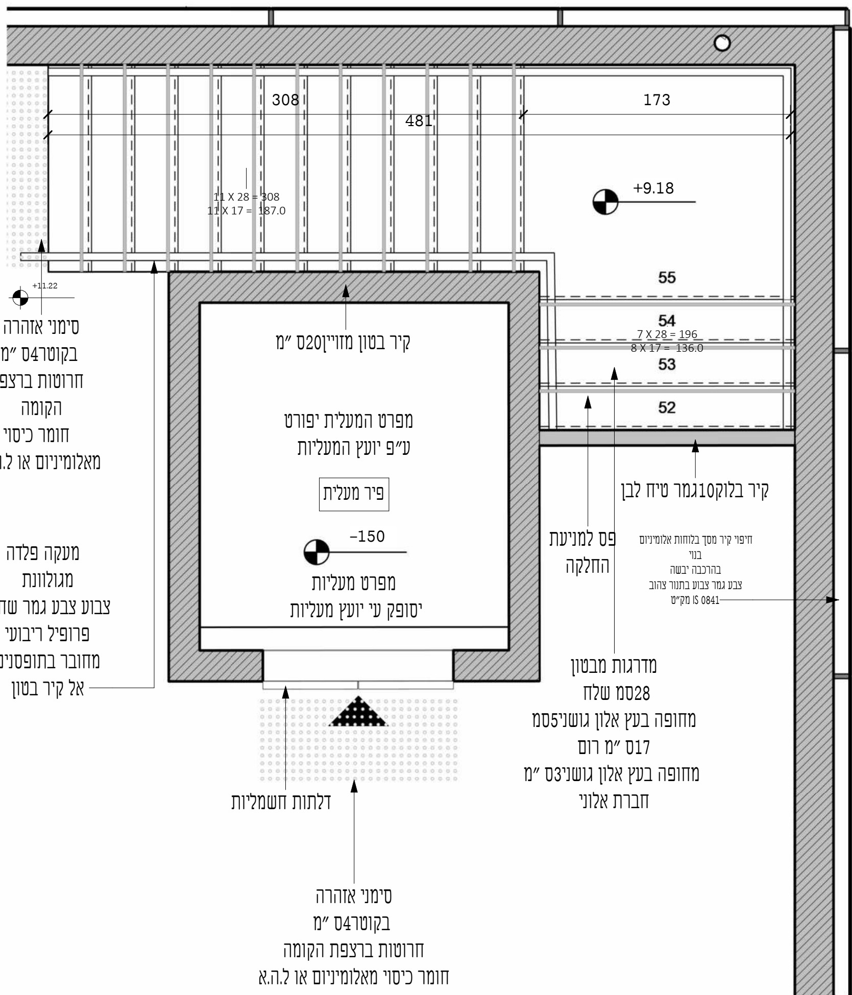
תוכנית מדרגות קומה ב' 1:25
