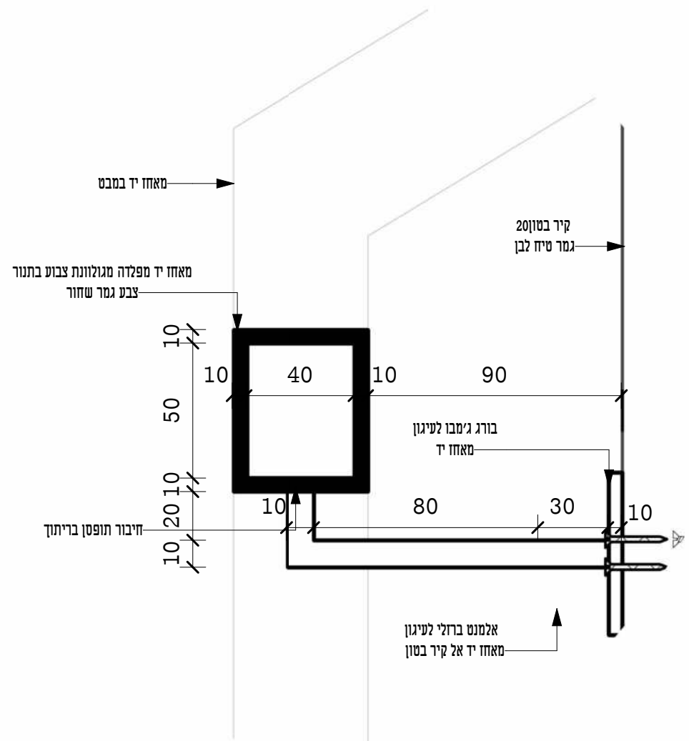
פרט מאחז יד 1:2
